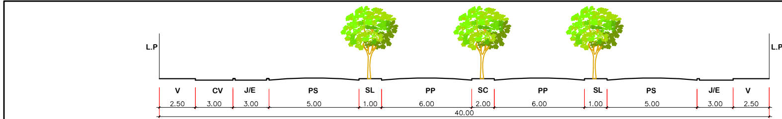
SECCIÓN A-A VIA ARTERIAL CON CICLOVIA NOMBRE: PANAMERICANA SUR
