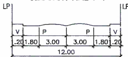
SECCION VIAL 2 - 2
