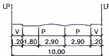
SECCION VIAL 3 - 3
