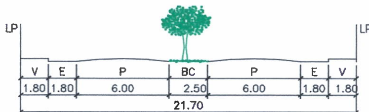
SECCION VIAL 1- 1
